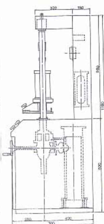
側面図
